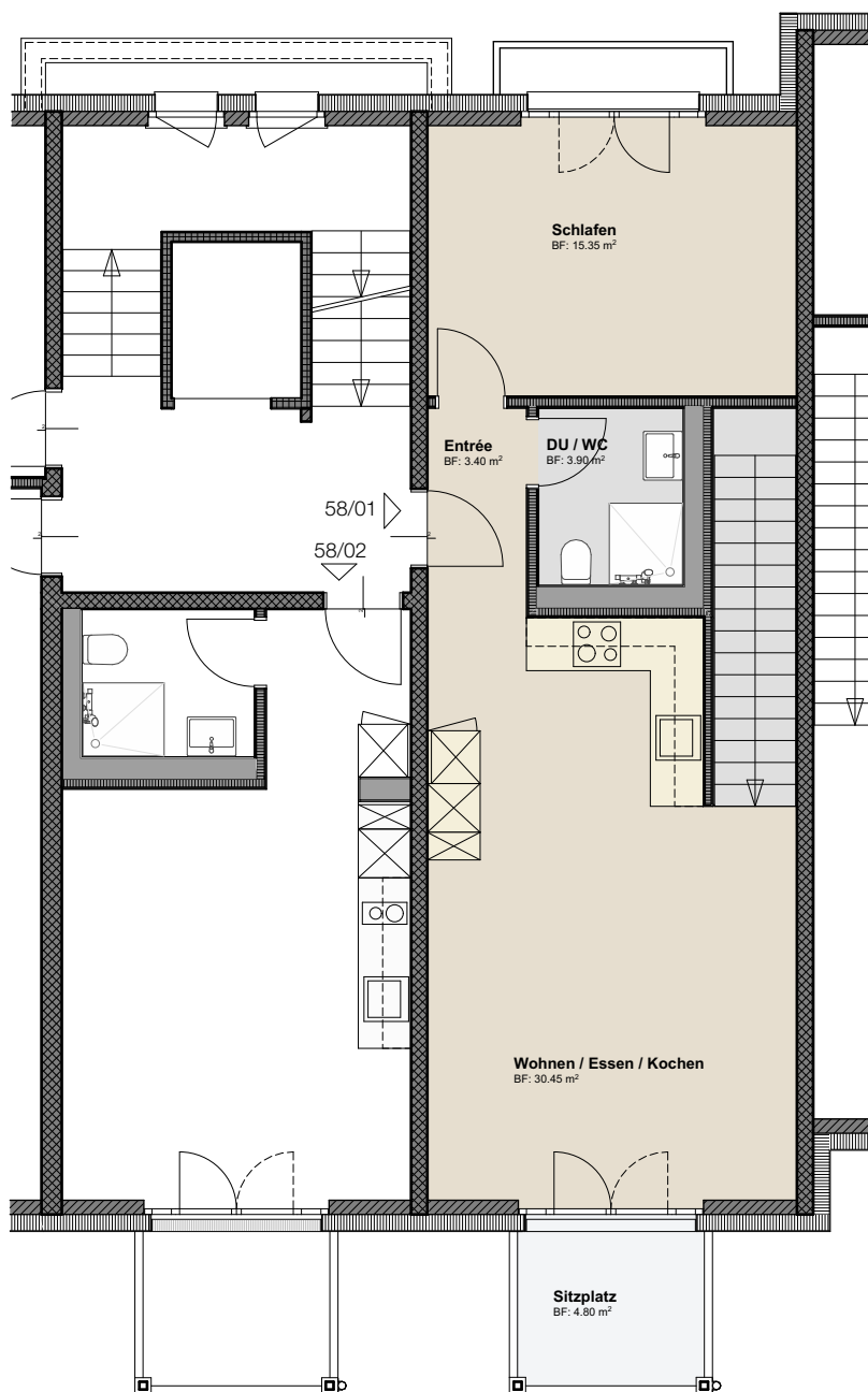
Erdgeschoss
