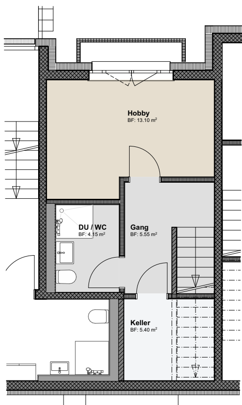
Sockelgeschoss
